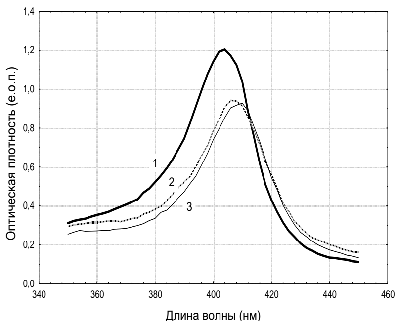
Рис. 3. График сравнения интегральных спектров 0.02%-ных растворов метгемоглобина: 1 – контрольный спектр интактного белка, 2 – спектр белка, контактирующего с хлороформом 3 – спектр белка, контактирующего с хлороформом под действием МП КНЧ.
